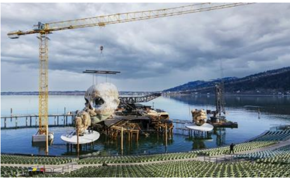
liebherr-150ecb-bregenz-03.jpg
