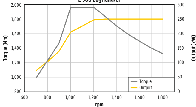
L 580 LogHandler
