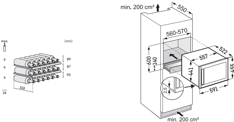
安装示意图
