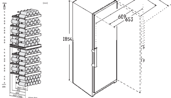
安装示意图
