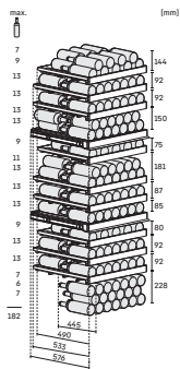
安装示意图
