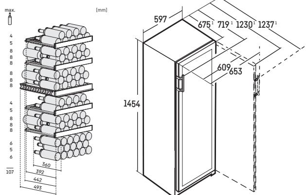
安装示意图
